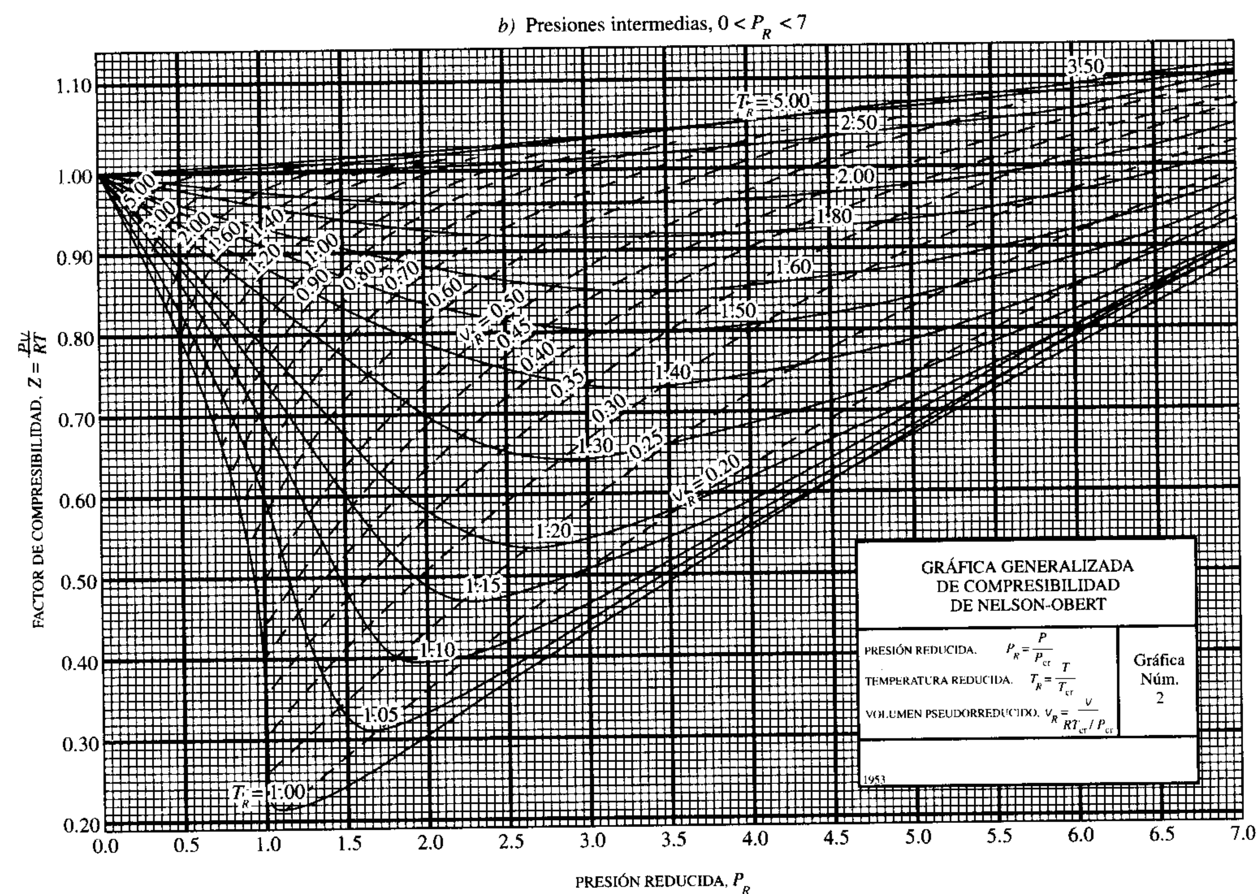
FIGURA A-15 Gráfica generalizada de compresibilidad de Nelson-Obert.
